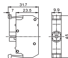
Schaltelemente und Lampenhalter B3...
