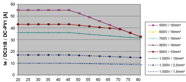
Schalter gekapselt LS55 PFL..., 2 Kontakte in Serie (A2)
