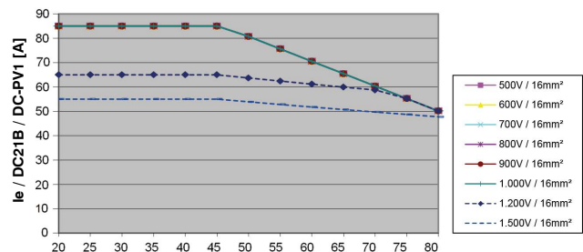
Schalter gekapselt LS55 PFL..., 4 Kontakte in Serie + 2 parallel (A4+2)
