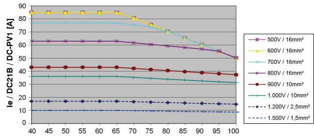
Schalter offen LS55 ..., 2 Kontakte in Serie + 2 parallel (A2+2)
