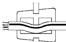
Blockierprinzip des Kabels
