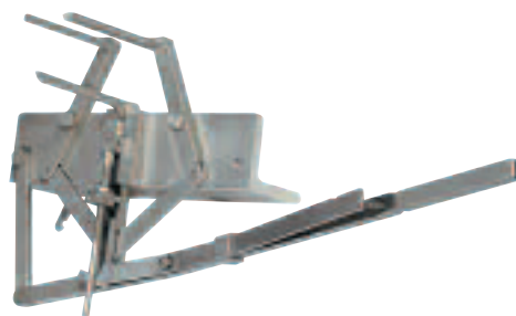
Aufweitwerkzeug zur Montage am Werkstisch D1/2-01
