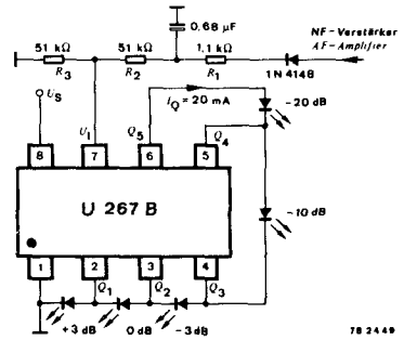
Fig. 4 Logarithmische NF-Aussteuerungsanzeige mit 5 LED's Logarithmic AF recording level display with 5 LED's
